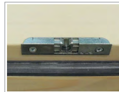
SCHNÄPPER Halter optional mit ETÖ, AV4D, EAV4, EAV4+ Verr. Oben montiert!
