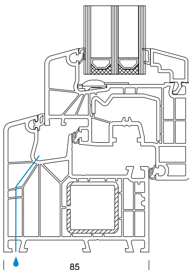
ENTWÄSSERUNG NACH UNTEN
