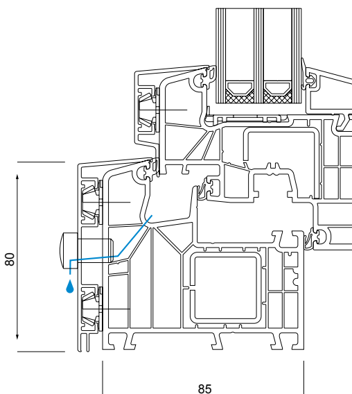
ENTWÄSSERUNG DURCH ALUSCHALE
